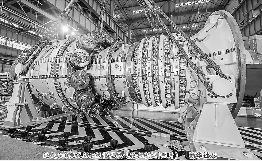
这是300兆瓦级F级重型燃气轮机（资料照片）。新华社发
